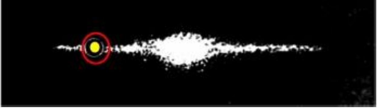
GALAXIA CALEA LACTEE văzută din lateral.
